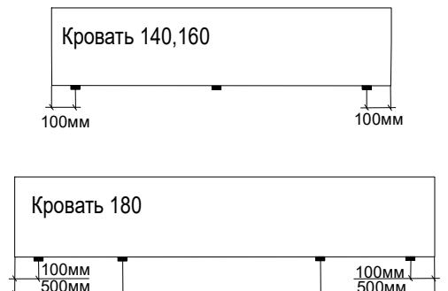
Схема установки подпятников
